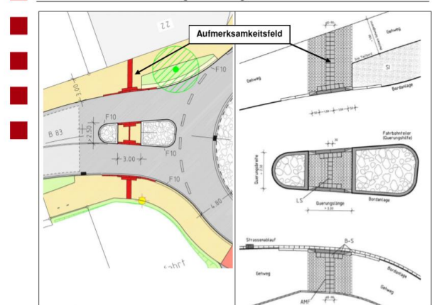
Abb. 15: Überquerungsstelle für Fußgänger mit Aufmerksamkeitsfeld und „Kasseler Rollbord“
